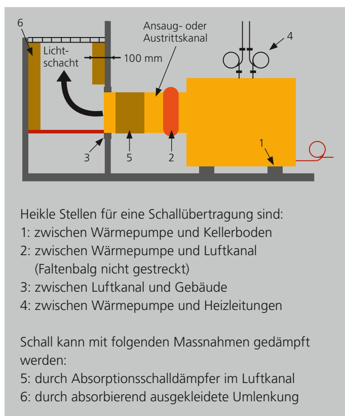
Lärminderungsmaßnahmen für eine Luft-Wasser-Wärmepumpe mit Luftansaugung über den Lichtschacht. Quelle: FWS
