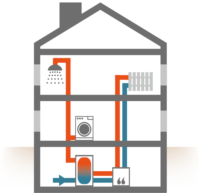
Warmwasserspeicher kombiniert mit Pelletheizkessel.
